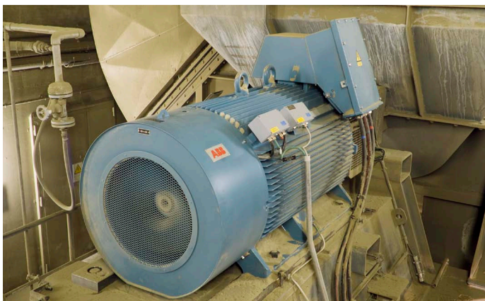
Der mit einem ACS 2000 von ABB drehzahlgeregelte Abluftgebläsemotor des Klinkerkühlers
